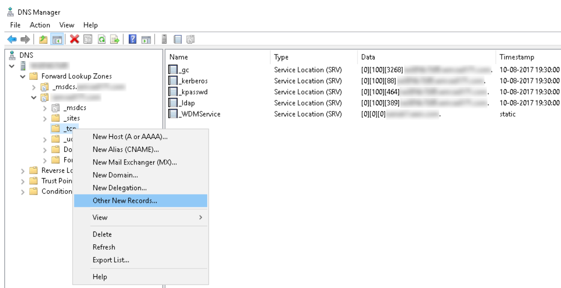
图 27: DNS 管理器
