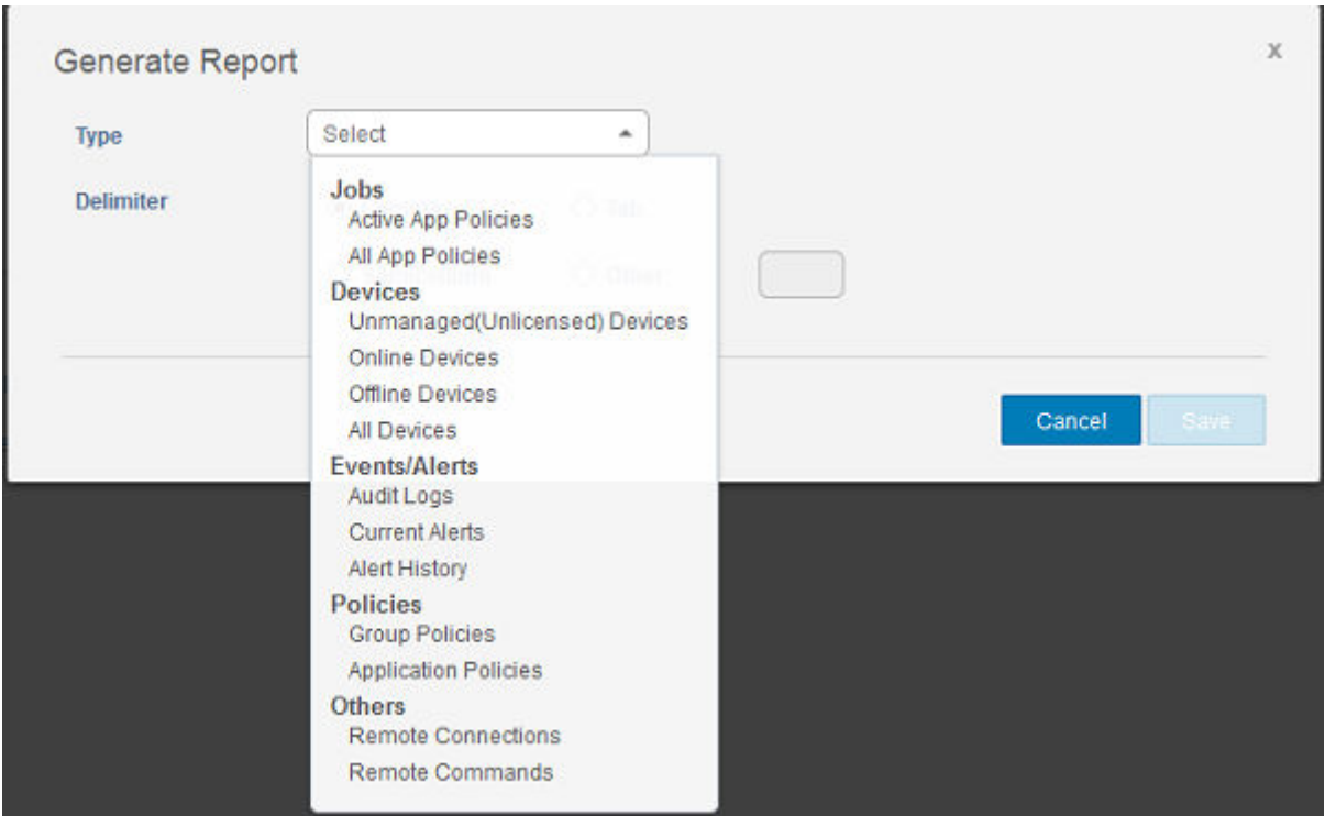
图 18: 报告类型
