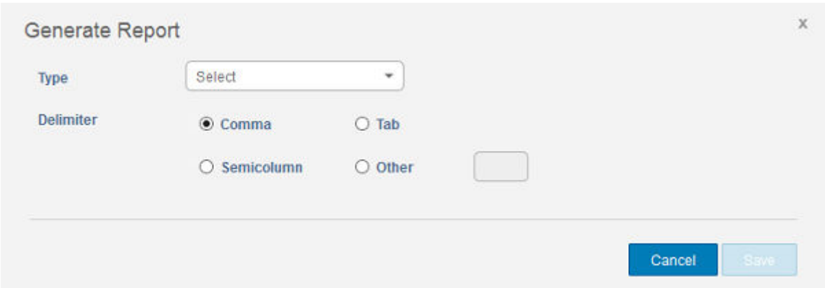
图 17: 生成报告
